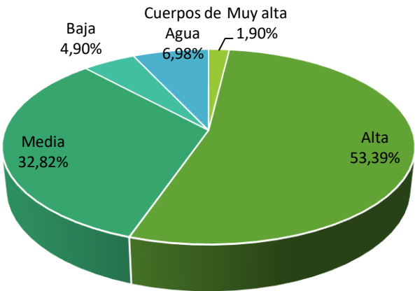
GRÁFICO 38. ZONAS SUSCEPTIBLES A EROSIÓN.
