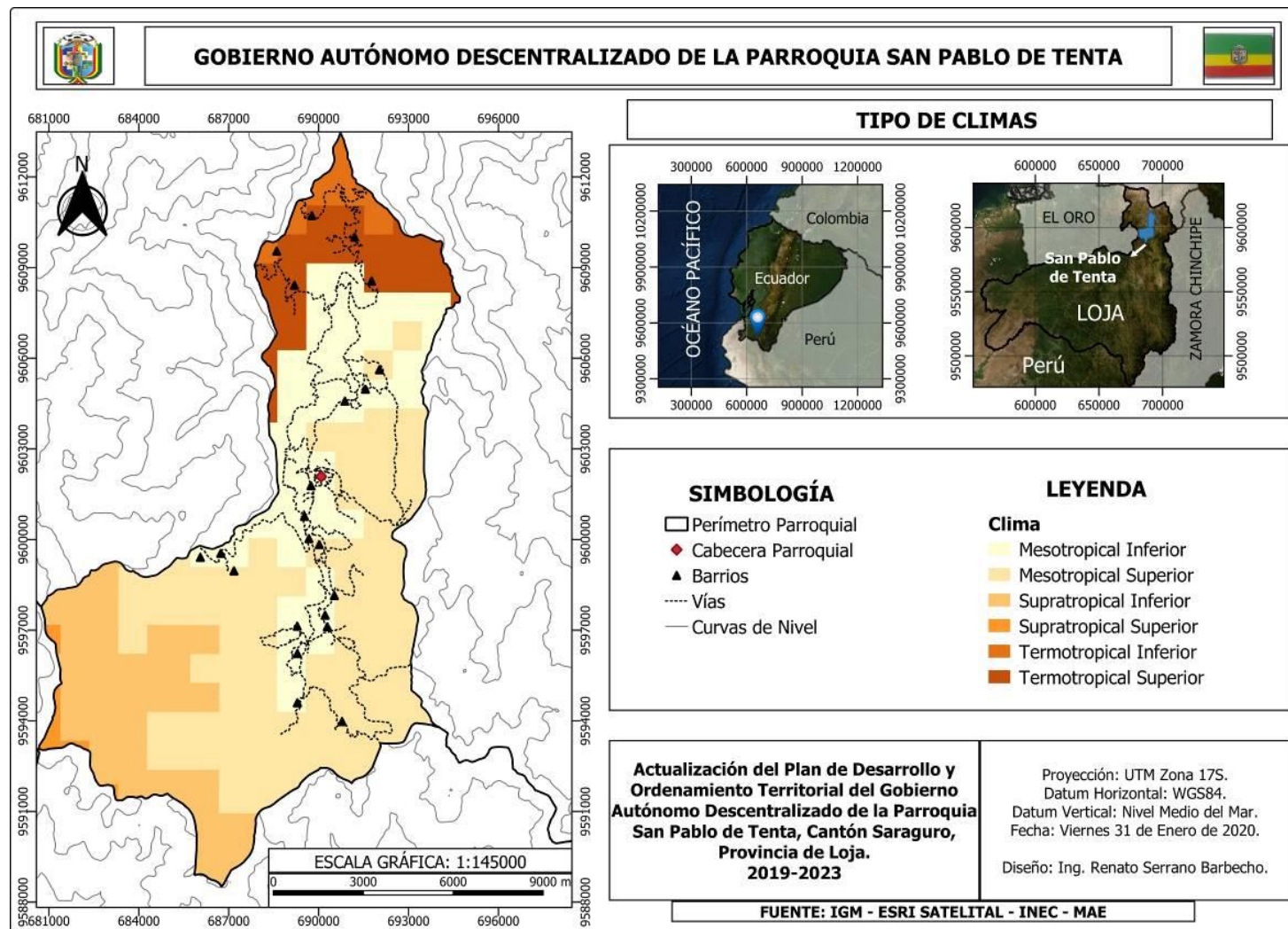
MAPA 17. TIPO DE CLIMAS DE LA PARROQUIA.
