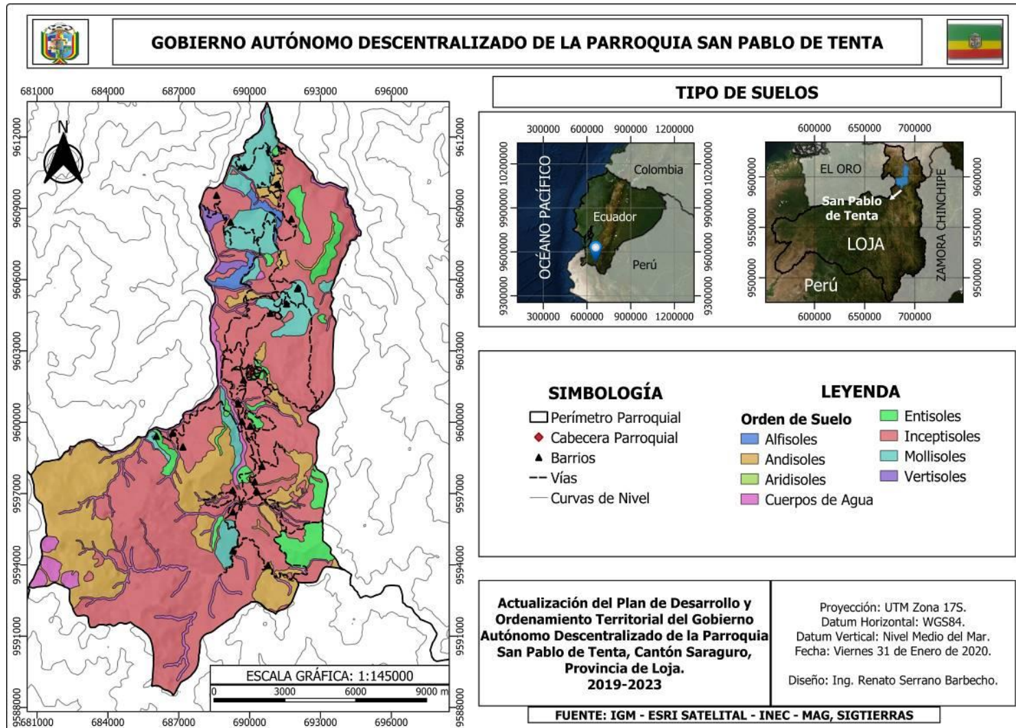
MAPA 11. TIPO DE SUELO DE LA PARROQUIA SAN PABLO DE TENTA.
