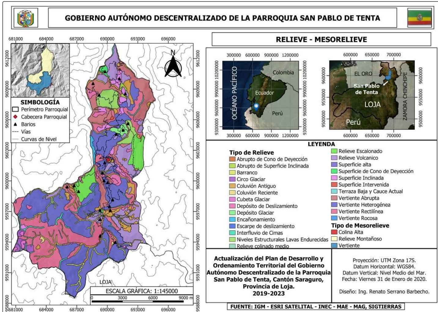
MAPA 6. GEOMORFOLOGÍA DE LA PARROQUIA.
