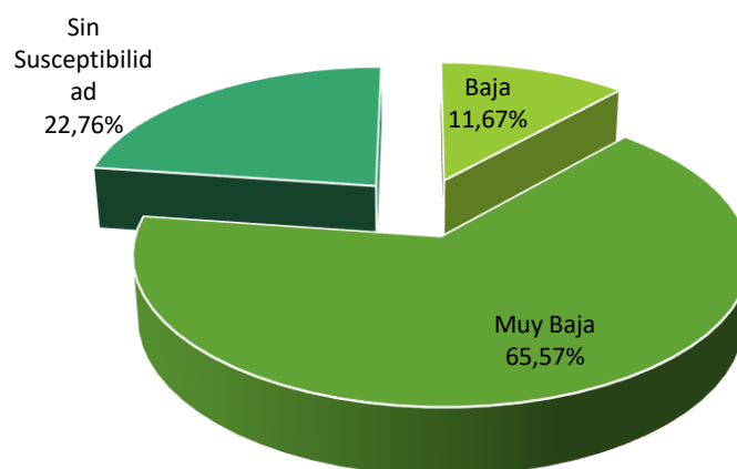
GRÁFICO 40. NIVEL DE SUSCEPTIBILIDAD A HELADAS EN LA PARROQUIA.
