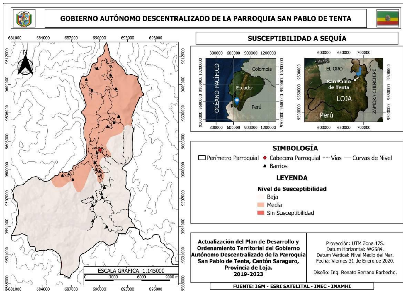
MAPA 26. NIVEL DE SUSCEPTIBILIDAD DE SEQUÍA EN LA PARROQUIA.
